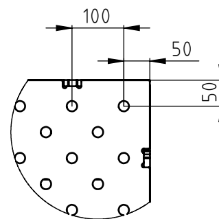
DETAIL A MĚŘITKO 1 : 10
